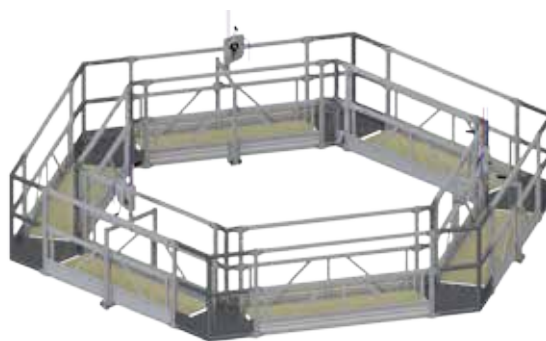
Plataforma compuesta por módulos de 2 m de longitud y piezas angulares de 60° con 3 elevadores manuales y liras de paso.
